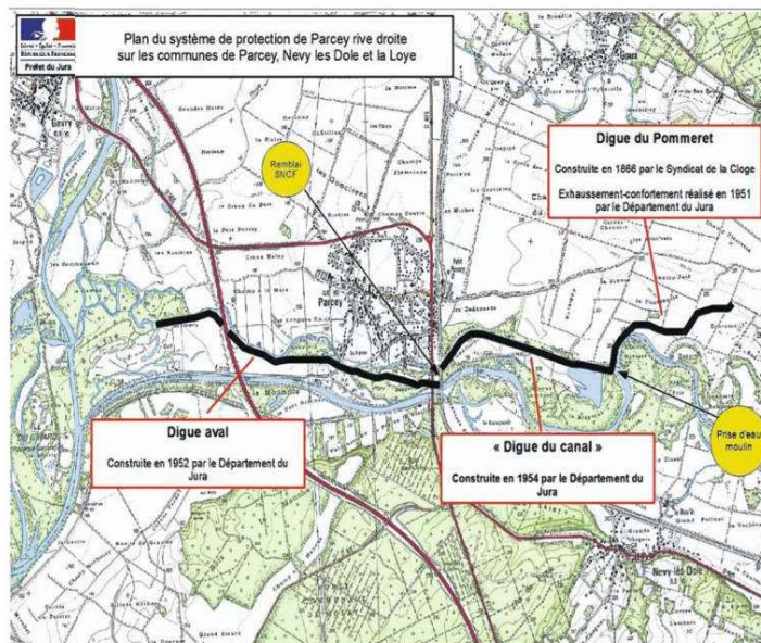
Parcey SNTH : plan des digues à Parcey (crédit SMDL)
